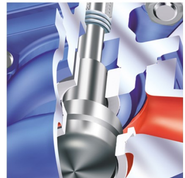
Посилена конструкція штока та направляюча
