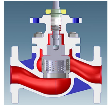
Багатоступенева редукція
