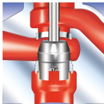
Триходові клапани із затвором, що змішує потоки
