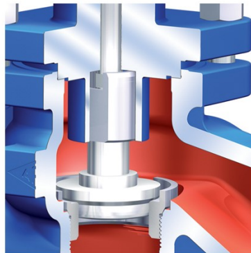
Змінні сідла
