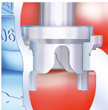
Шліцьовий затвор Підвищені перепади тиску
