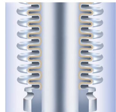
Двошаровий сальфон із н/ж сталі (опція)
