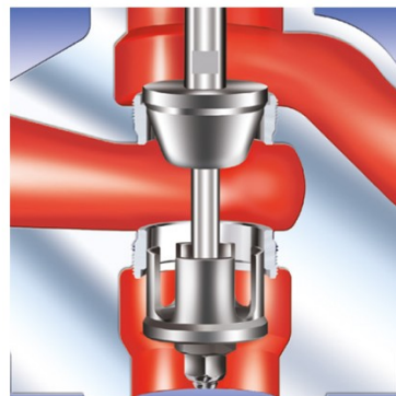
Триходові клапани із затвором, що розділяє потоки
