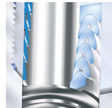
V - подібні кільця сальників з PTFE Динамічне сальникове ущільнення штока
