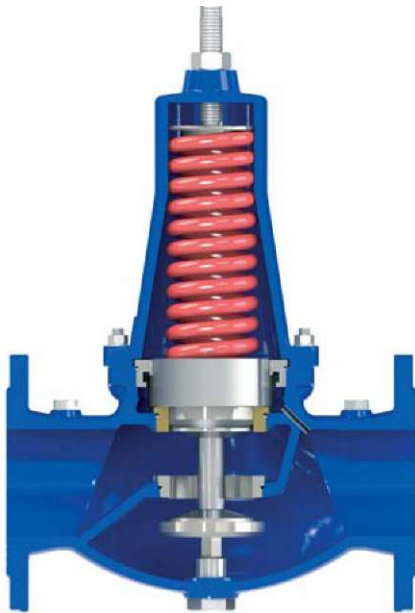
Клапан нормально відкритий
