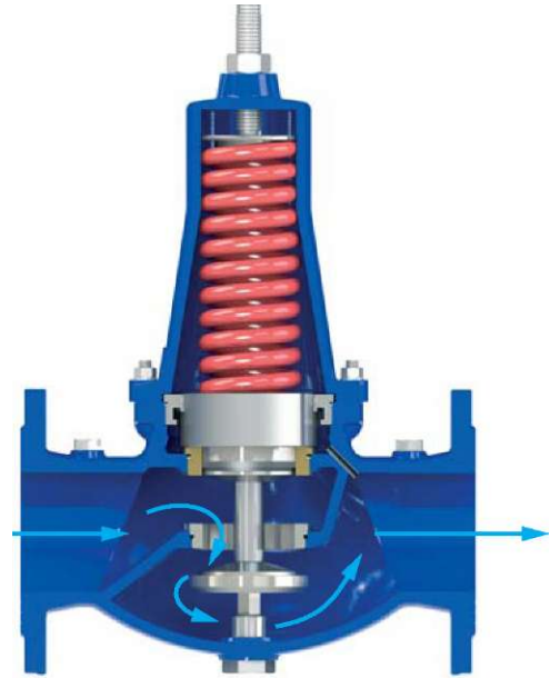
Клапан повністю відкритий
