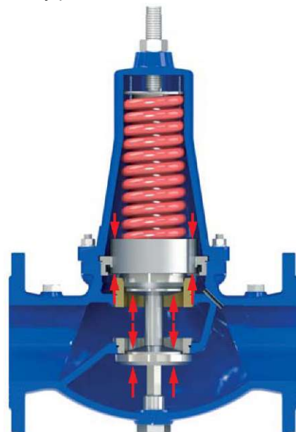
Клапан повністю закритий (статичні умови)
