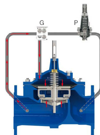
Закриття клапана
