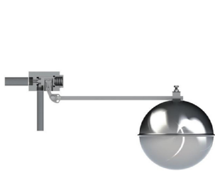
Модель MCP
